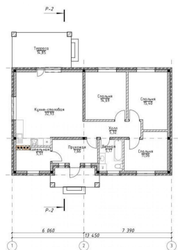
План первого этажа М1:100
