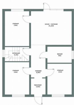
Этаж 1 Вариант 2, лестница в техническом помещении
