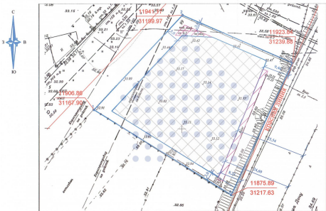
Чертеж градостроительного плана земельного участка М 1:500
